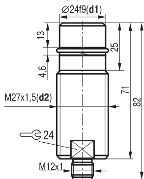
Схема монтажа
